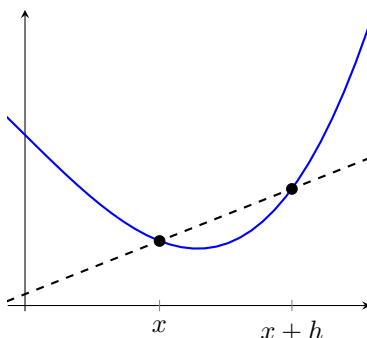
Figur 48: Sekant—den rätta linjen genom punkterna (x, f(x)) och (x + h, f(x + h)) .
