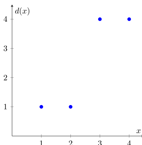
Figur 6: Grafen till funktionen d i Exempel 3.2.3.
