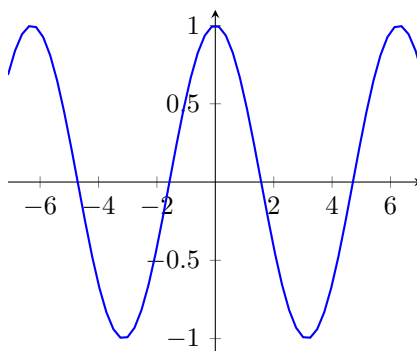
Figur 35: Grafen till funktionen f(v) = \cos v på intervallet [-2\pi, 2\pi] .
