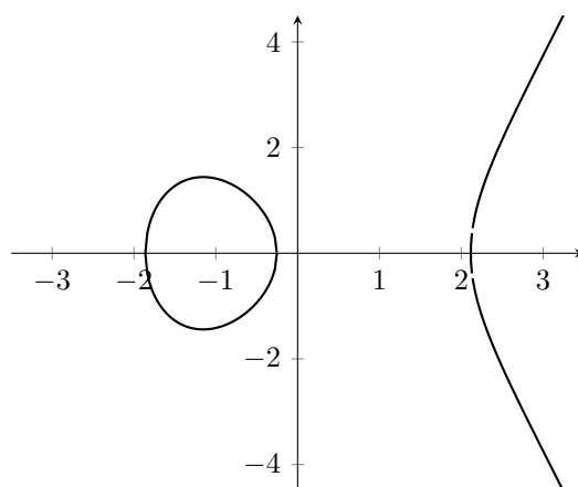
Figur 16: Den elliptiska kurvan y^2 = x^3 - 4x - 1 på intervallet [-3, 3] .
