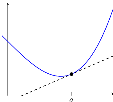
Figur 47: Grafen till en funktion samt dess tangent (den rätta linjen) i en punkt.
