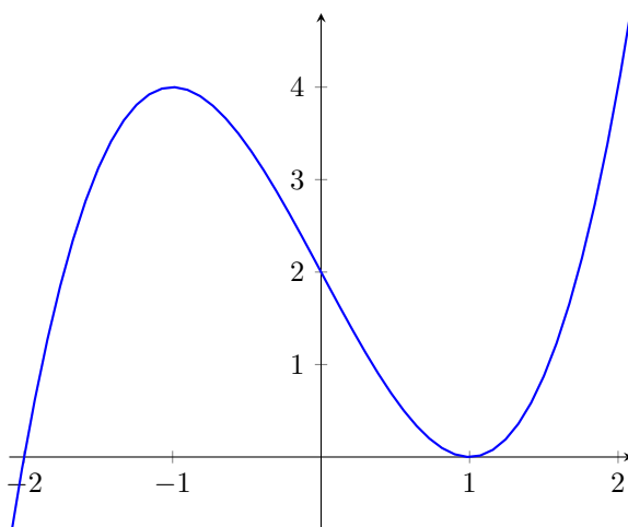
Figur 53: Skiss av grafen y = x^3 - 3x + 2 .
