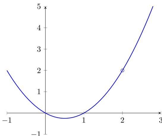
Figur 45: Grafen till h(x) = \frac{x^3 - 3x^2 + 2x}{x - 2} , vilken sammanfaller med grafen för p(x) = x(x - 1) = x^2 - x i alla punkter utom x = 2 . När x = 2 är h(x) inte definierad. Då x går mot 2 går funktionen mot värdet 2.
