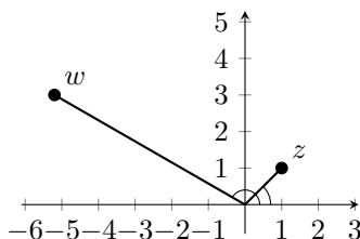
Figur 42: Punkten z = 1 + i samt w = -3 + 4i det komplexa talplanet.
